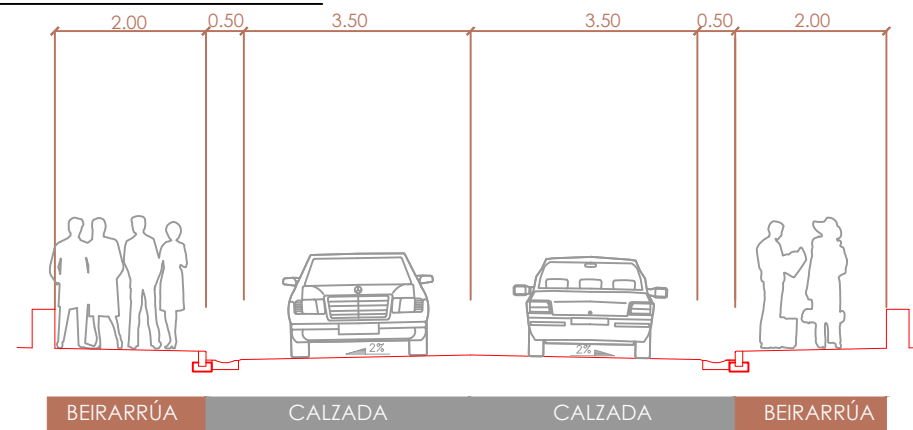
SECCIÓN A1-A1
