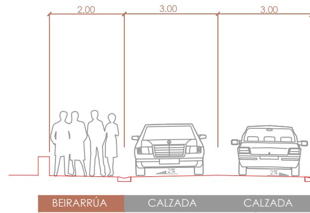
SECCIÓN B1-B1
