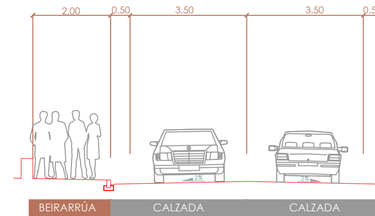
SECCIÓN D-D
