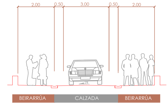
SECCIÓN A2-A2
