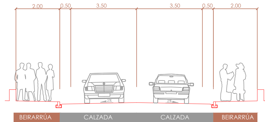
SECCIÓN C-C
